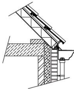
Detail 100.12
