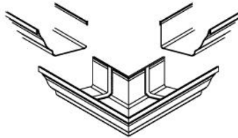
Detail 100.12
