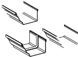
Detail 100.03 Verbindingsstuk
